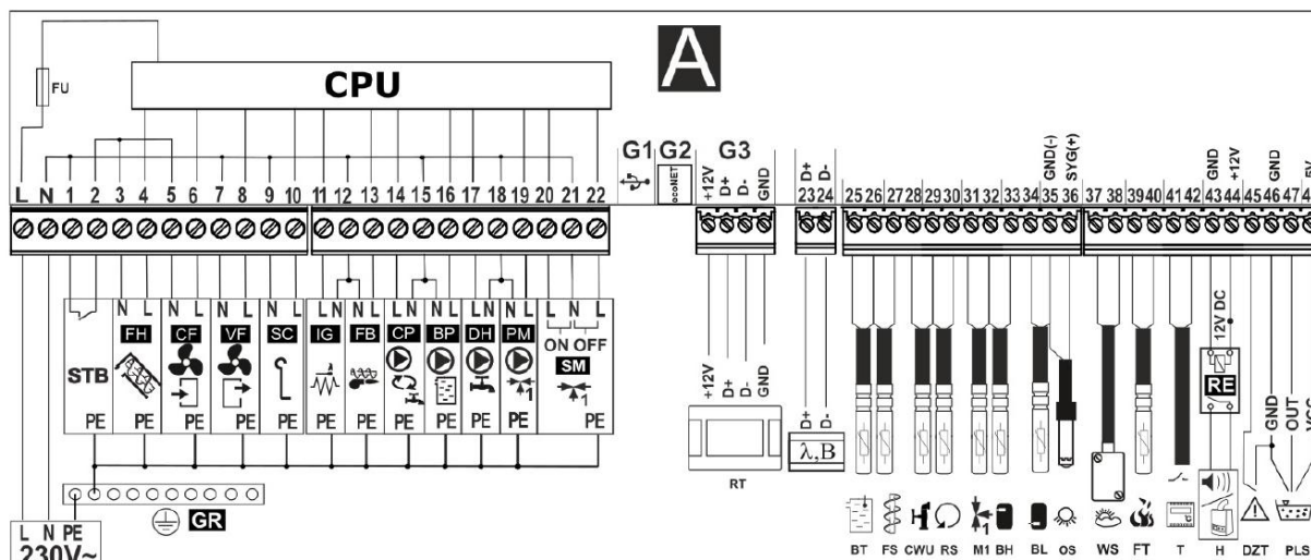
Rysunek 22 - Schemat połączeń elektrycznych regulatora L N PE -zasilanie sieciowe 230V ~, CPU -sterowanie, FU -bezpiecznik, STB -wejście do ogranicznika temperatury bezpieczeństwa, FH -podajnik główny, CF -wentylator nadmuchiowy palnika, VF -wentylator wyciągowy, SC -silnik obrotowy czyszczenia palnika, IG -zapalarka, FB -podajnik palnika, CP -pompa cyrkulacji CWU, BP -pompa kotła, DH -pompa CWU, PM -pompa mieszacza 1, SM -siłownik mieszacza 1, RT -panel pokojowy ecoSTER TOUCH z funkcją termostatu pokojowego, λ -moduł sondy Lambda, B -moduł do obsługi dodatkowych obiegów grzewczych, BT -czujnik temperatury kotła typu CT4, FS -czujnik temperatury podajnika typu CT4, CWU -czujnik temperatury CWU typu CT4, RS -czujnik temperatury wody powracającej do kotła typu CT4, M1 -czujnik temperatury obiegu regulowanego (mieszacza 1) typu CT4, BH -czujnik temperatury bufora górny typu CT4, BL -czujnik temperatury bufora dolny typu CT4, OS -optyczny czujnik jasności płomienia, WS -pogogowy czujnik temperatury typu CT6-P, FT -czujnik temperatury spalin typu CT2S, T -termostat pokojowy (zwierno-rozwierny), H -wyjście napięciowe do sterowania kotłem rezerwowym R lub do sygnalizacji alarmów AL, RELAY -przełącznik 12VDC, DZT -czujnik otwarcia drzwi kotła lub klapy zasobnika, PLS -czujnik poziomu paliwa
