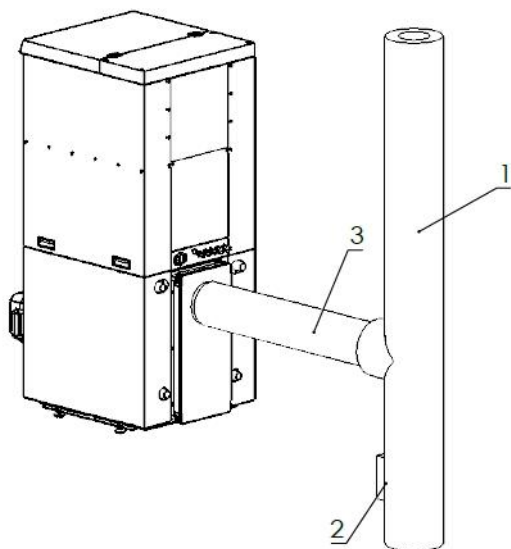
Rysunek 14 - Podłączenie do instalacji kominowej – proste 1 – Przewód kominowy; 2 – Wyczystka kominy; 3 – Zaizolowane podłączenie do kominy
