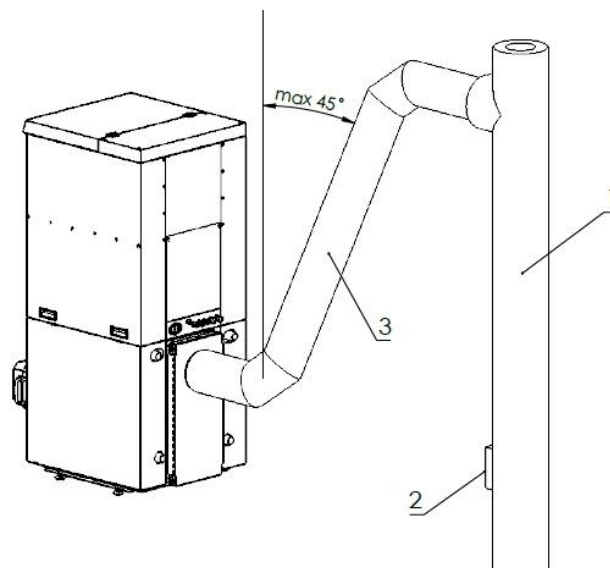
Rysunek 15 - Podłączenie do instalacji kominowej – pochylone 1 – Przewód kominowy; 2 – Wyczystka kominy; 3 – Zaizolowane podłączenie do kominy
