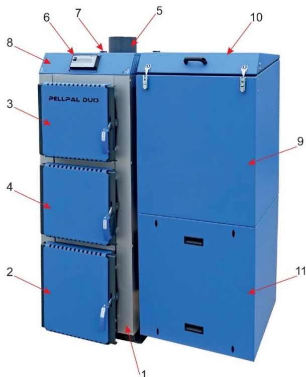
Rysunek nr 2a. Widok ogólny kotłów PELLPAL®DUO 18/24
