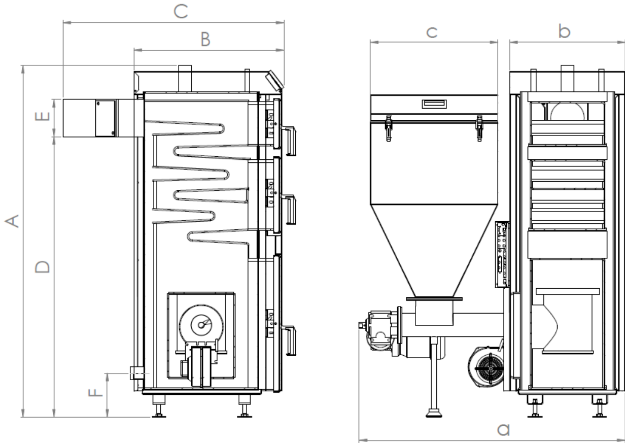
Rys.nr 1. Kocioł TORET - I 19kW, TORET 50kW
