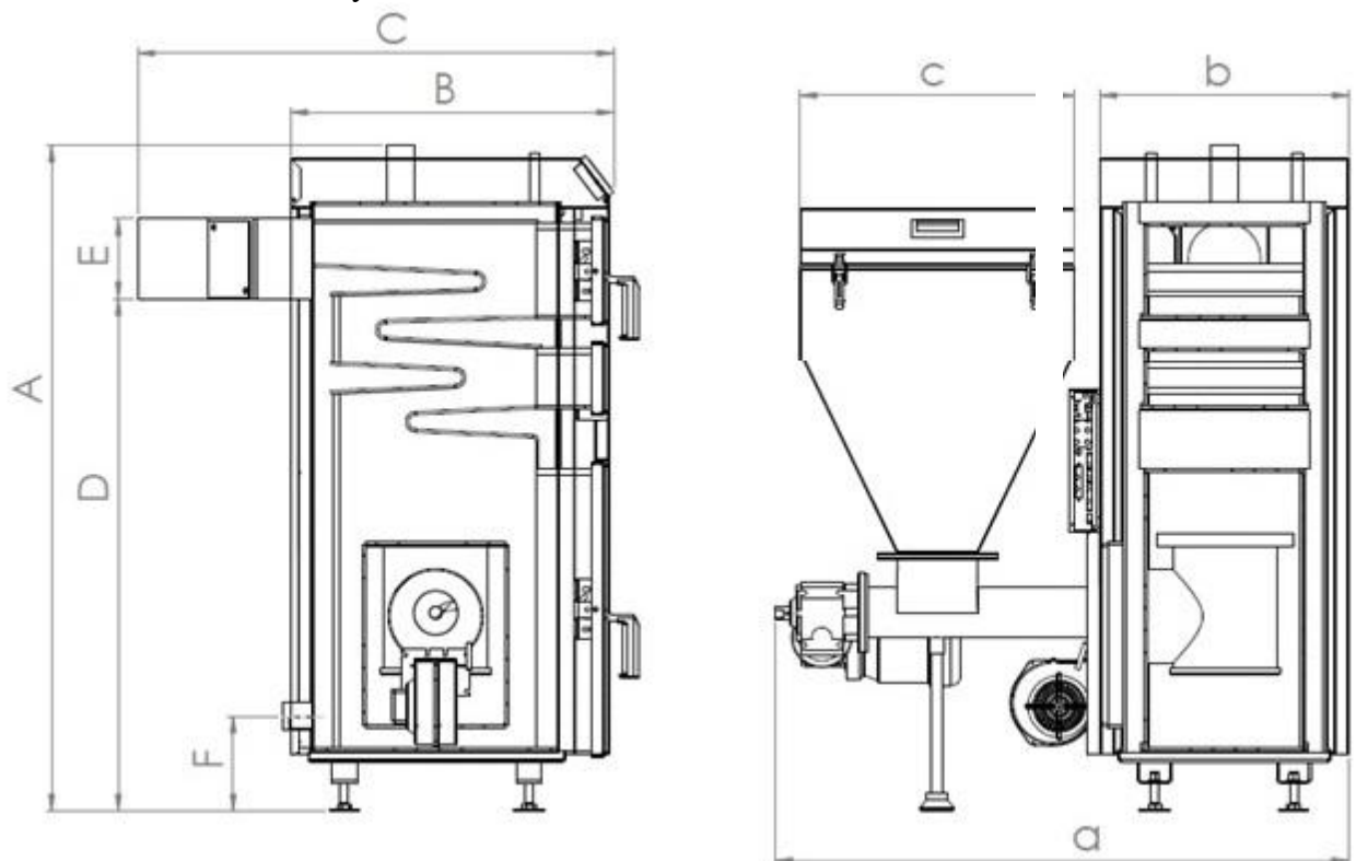
Rys.nr 2 Kocioł TORET -12kW
